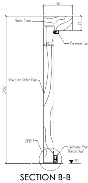
TIMBER DOOR FRAME
