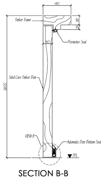
TIMBER DOOR FRAME
