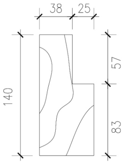
TIMBER DOOR FRAME
